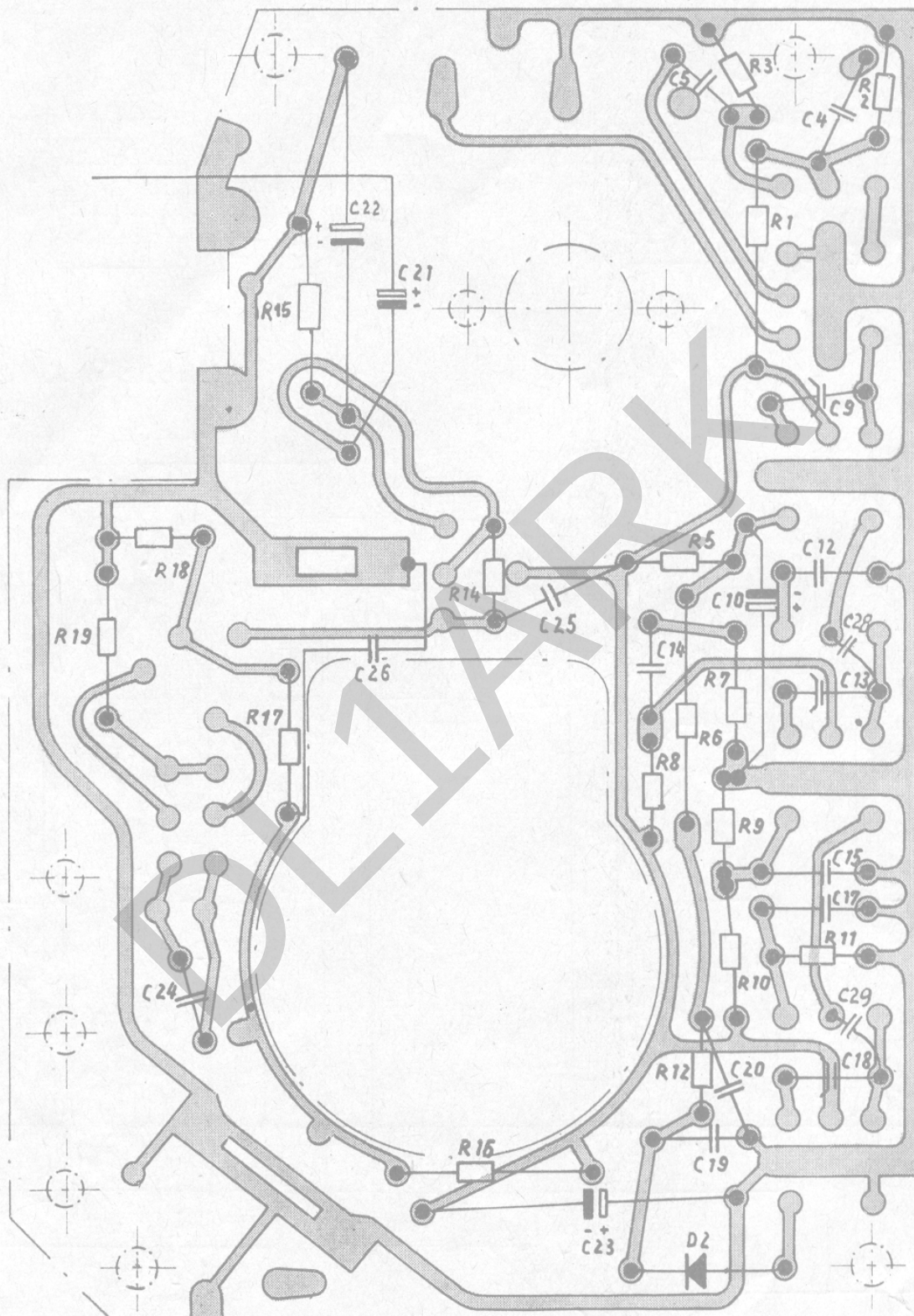
Schematische Darstellung der Anordnung von Kondensatoren u. Widerständen
